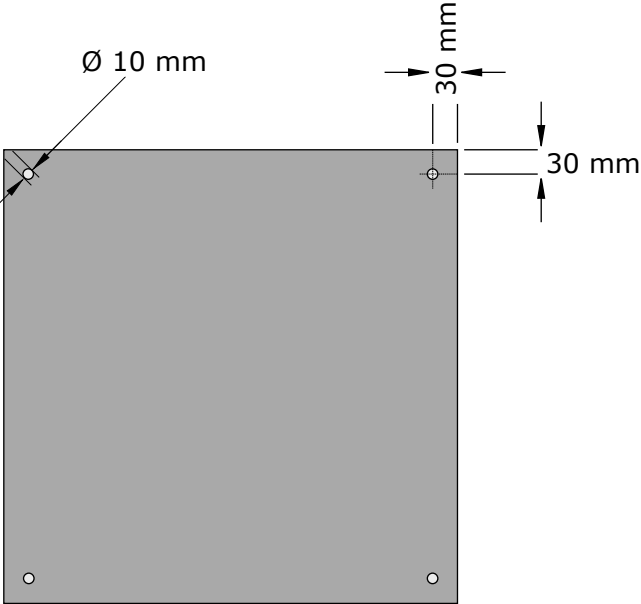
PLANTA
